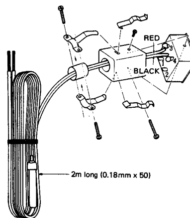
Fig. 16 DC cable
